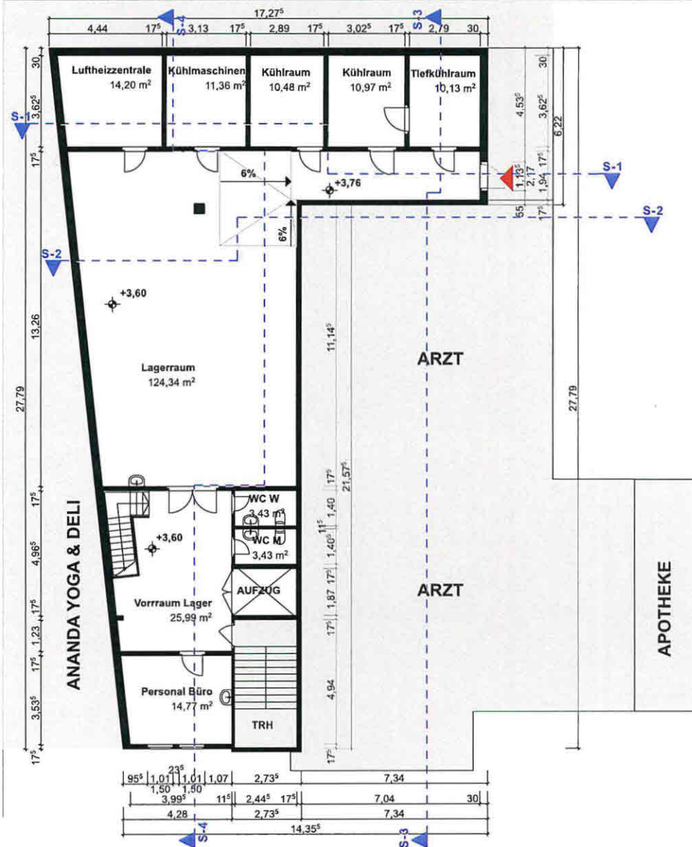
1. Obergeschoss Bestandsplan 1:100
