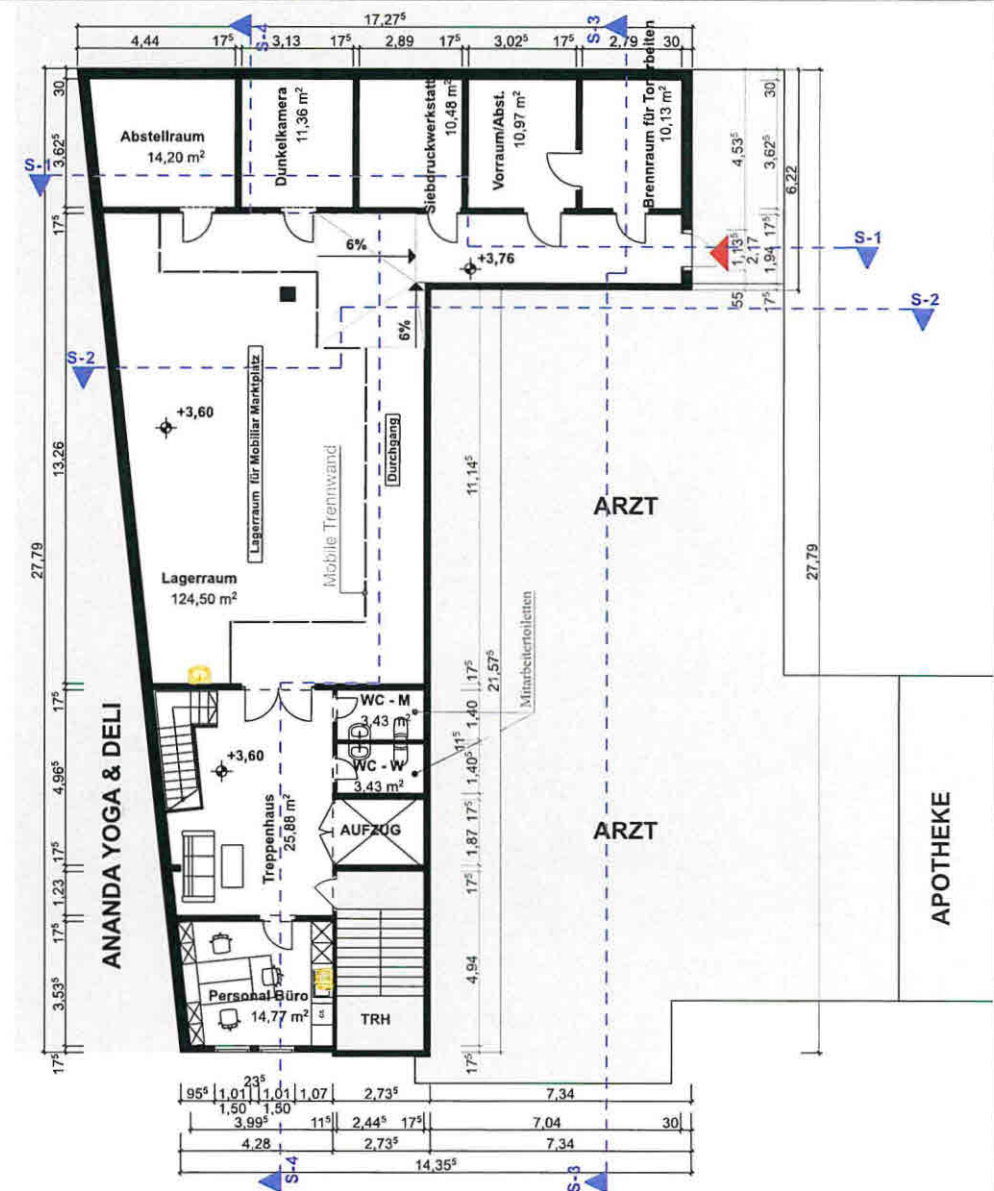
1. Obergeschoss Neuplanung 1:100
